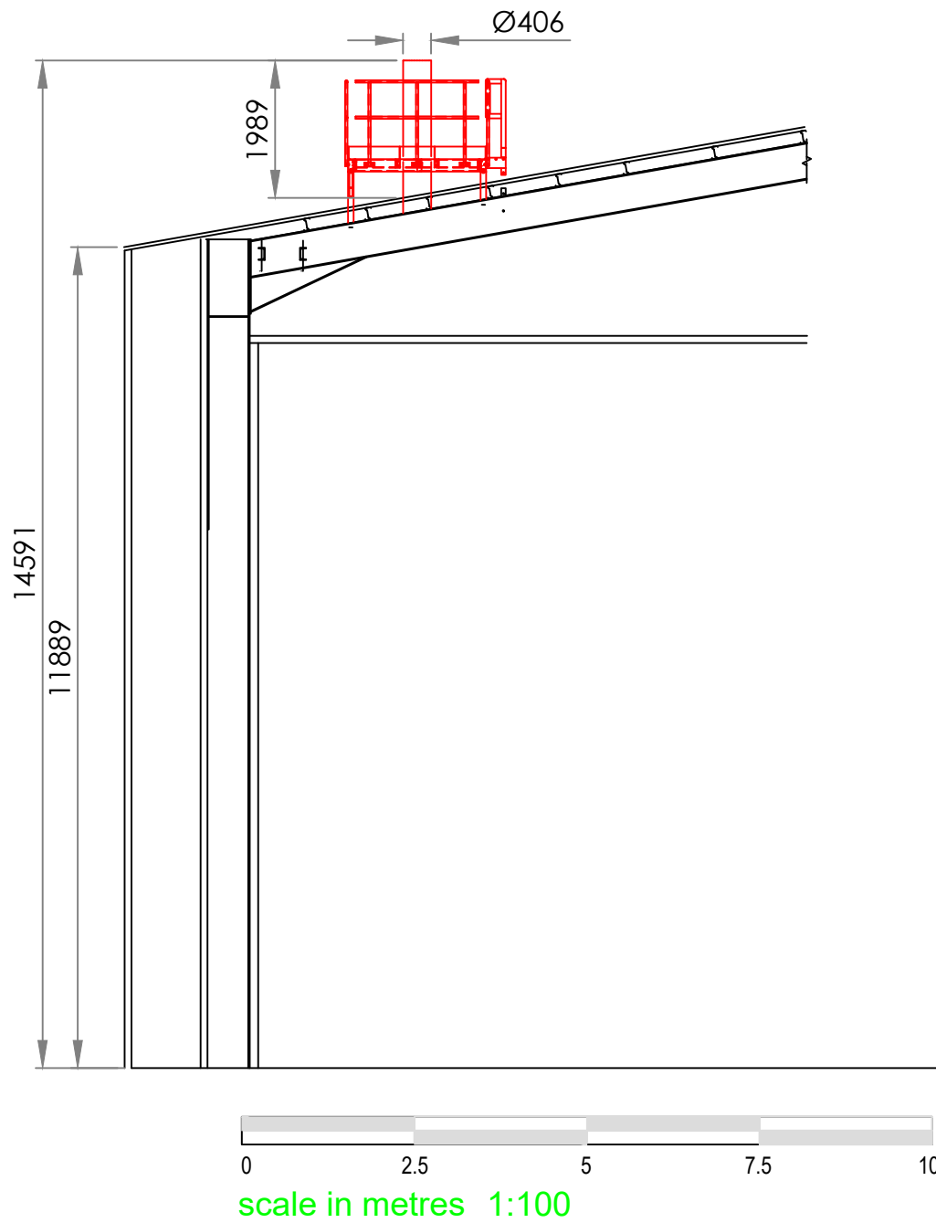
SECTION A-A
