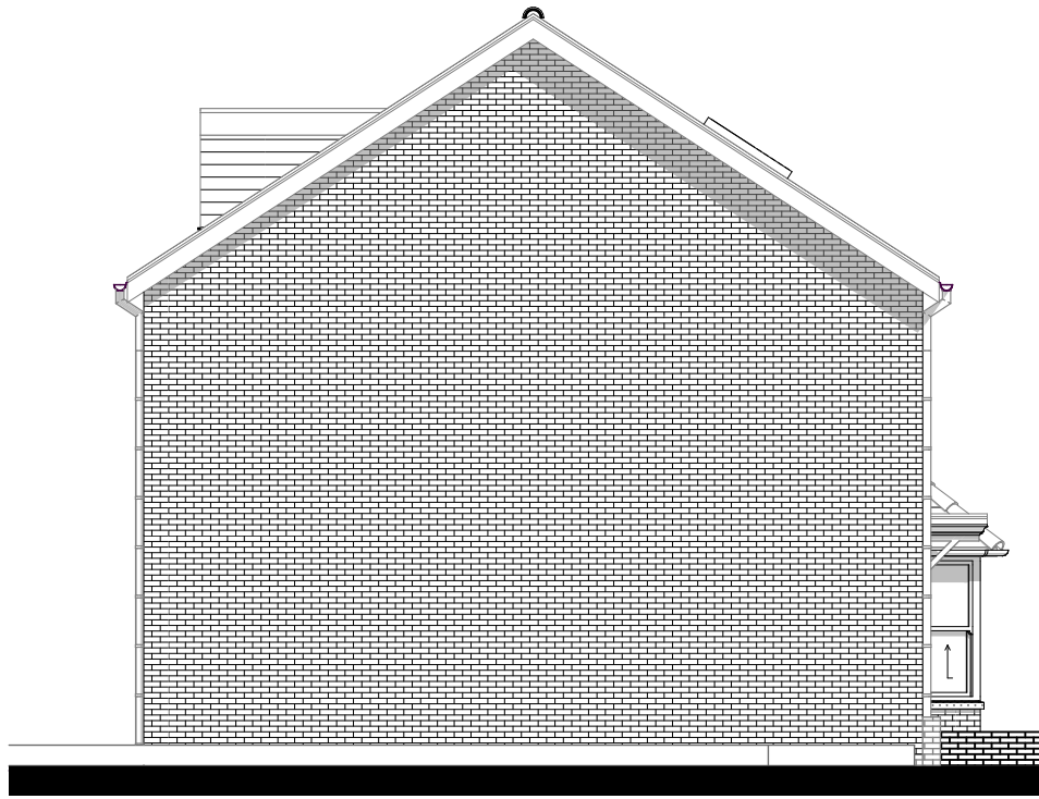
Flank Elevation
